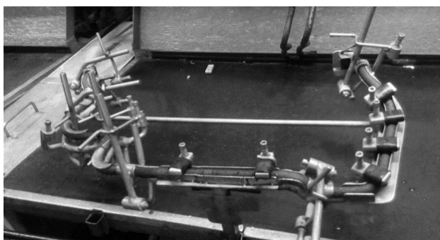
Zdjęcie 3. Forma z umieszczonym wewnątrz przewodem poliamidowym Źródło: E. Piecuch – opracowanie własne.
